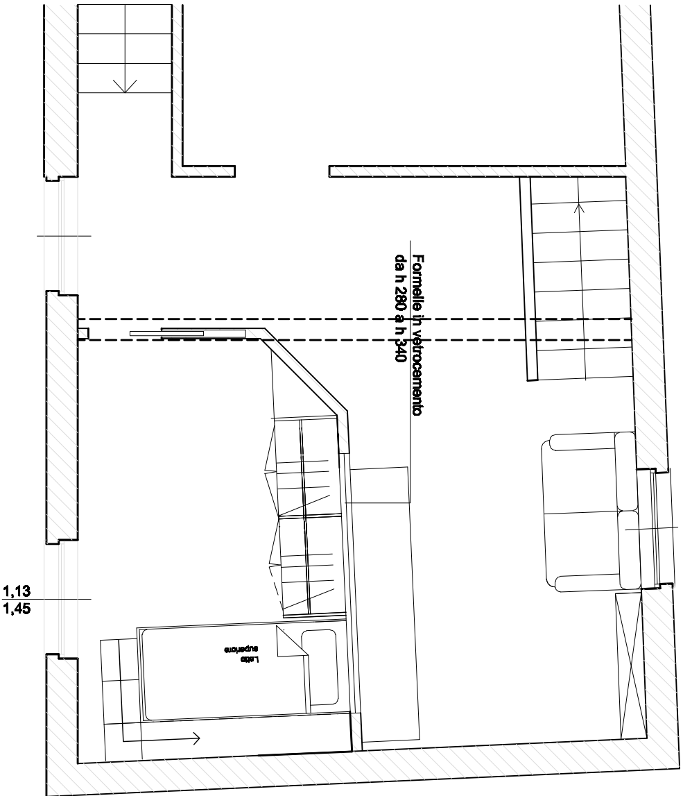
PIANTA PIANO PRIMO - STATO DI PROGETTO SOLUZIONE N.2
