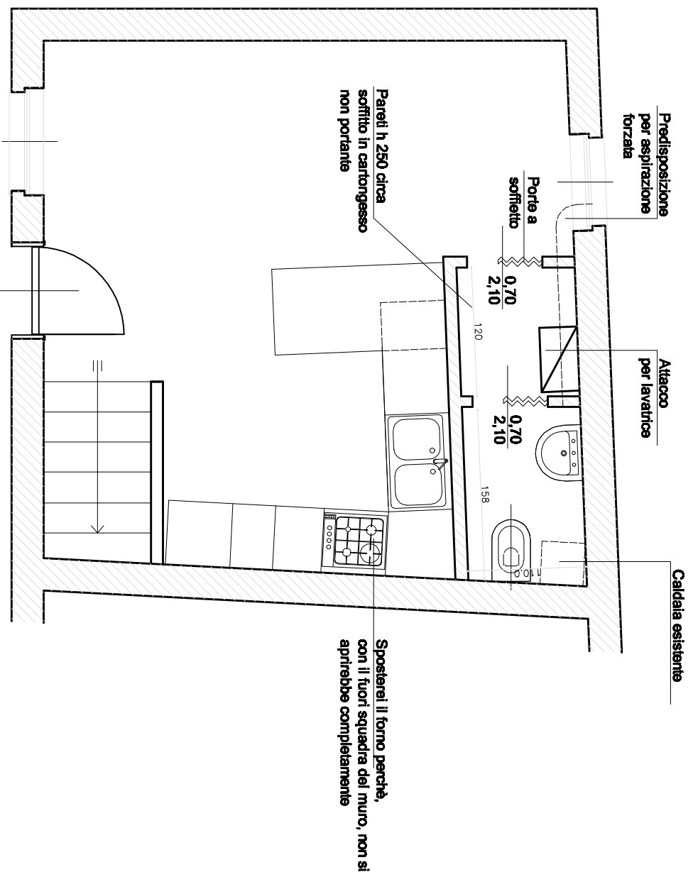
PIANTA PIANO TERRA - STATO DI PROGETTO
